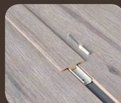
h 11,1 x w 44 x l 2400 mm T-Profile MDF
